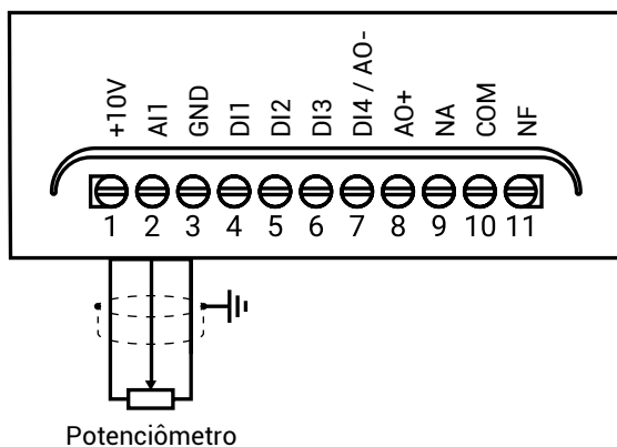
Figura 3.3.10 - Esquema de ligação do potenciômetro.
