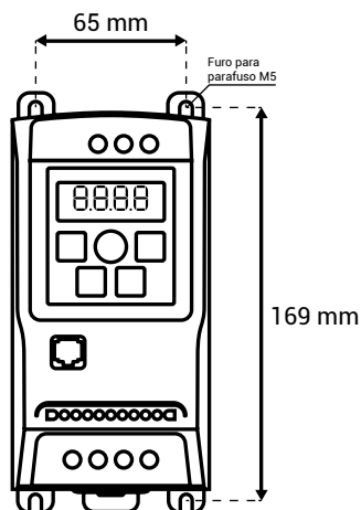
Figura 3.2.2. Dimensões mínimas para instalação mecânica.
