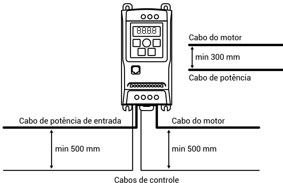
Figura 3.3.3 - Boas práticas para passagem dos cabos.
