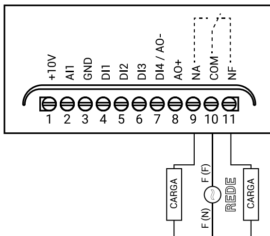
Figura 3.3.9 - Saída a relé.
