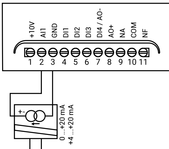
Dispositivo com fonte de alimentação elétrica isolada
