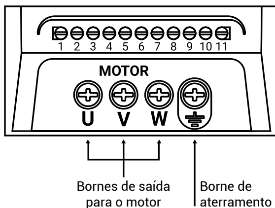
Figura 3.3.6 - Alimentação do motor.
