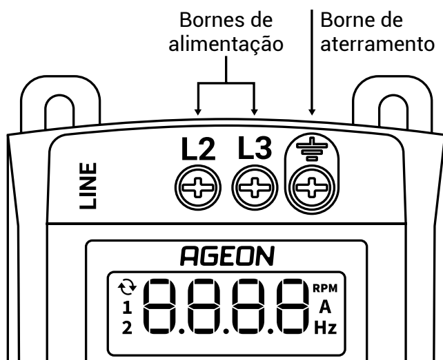
Figura 3.3.5 - Alimentação do inversor.
