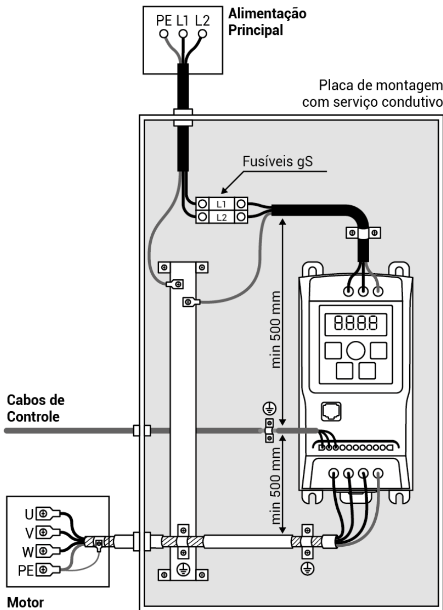
Figura 3.3.4 - Boas práticas para instalação em painel elétrico
