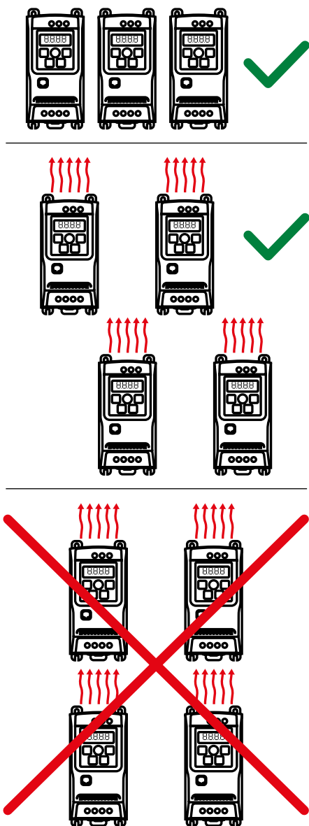
Figura 3.2.5. Boas práticas para instalação mecânica.
