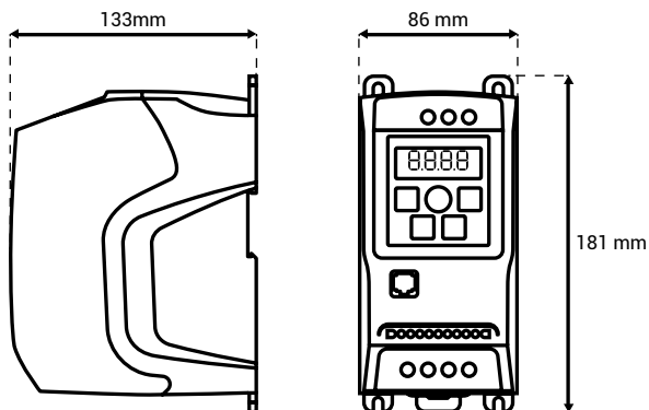
Figura 3.2.1. Dimensões do produto.
