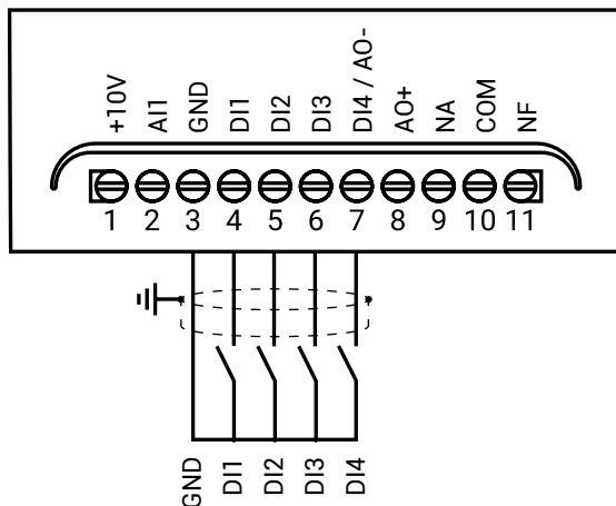
Figura 3.3.8 - Exemplo de ligação das entradas digitais.
