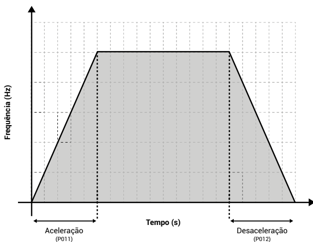
Figura 4.2.1 - Perfil de aceleração/desaceleração.
