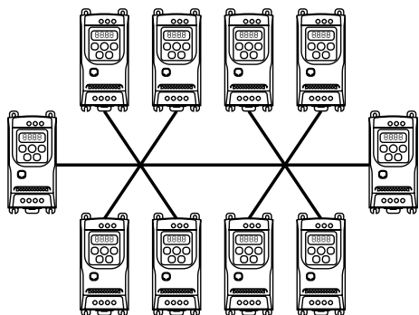
Barramento com estrelas (inadmissível)
