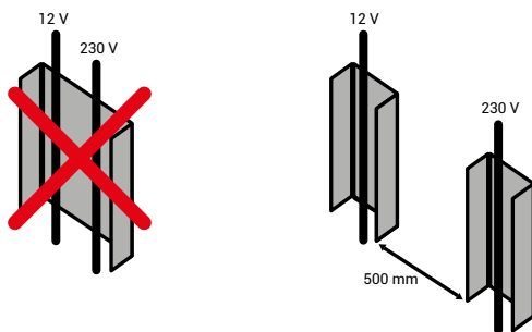
Figura 3.3.2 - Boas práticas para calhas de passagem de cabos.
