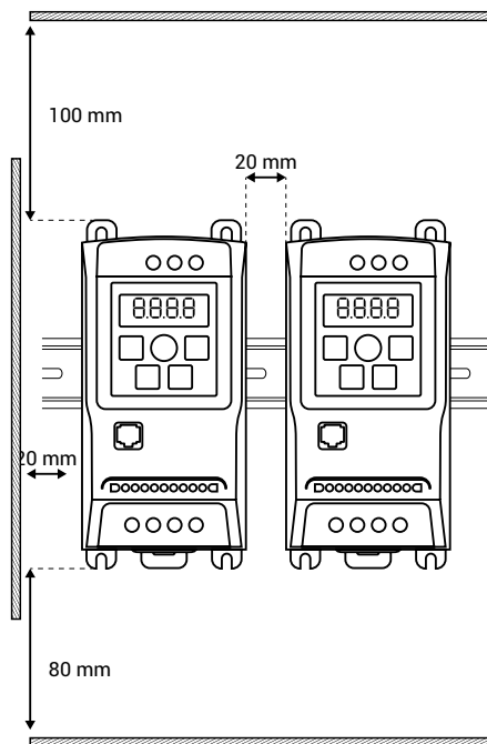
Figura 3.2.4. Detalhe para fixação no trilho DIN35.
