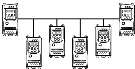
Barramento com derivações (tolerável)
