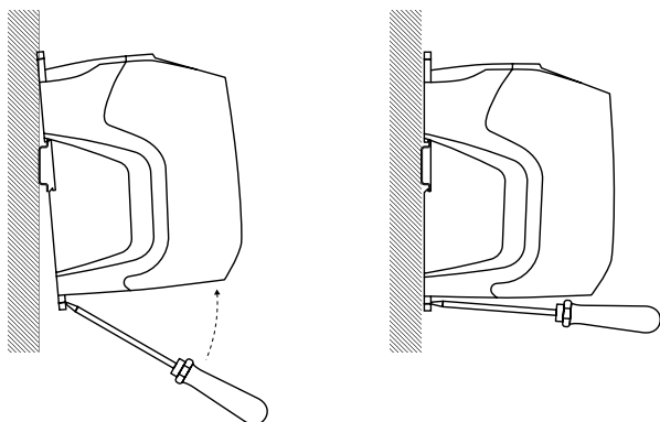
Figura 3.2.3. Detalhe para fixação no trilho DIN35.
