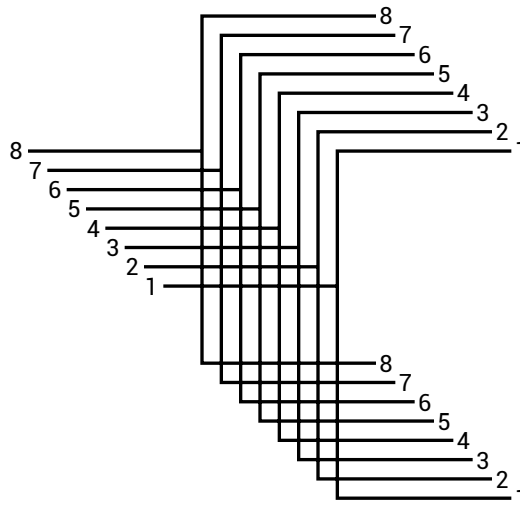
Figura 5.1.2. Ligação do adaptador Y.
