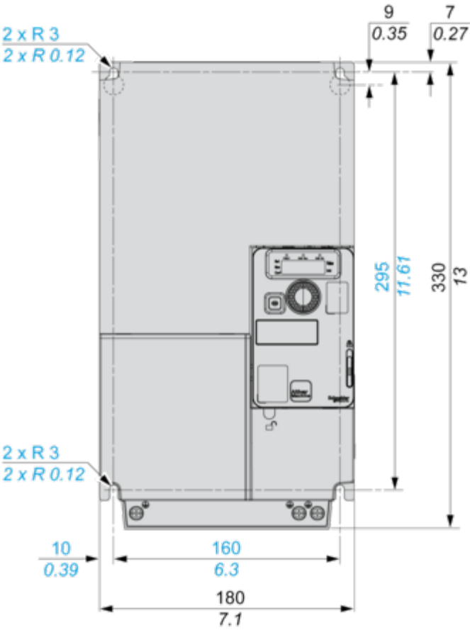
Vista direita e frontal com placa EMC
